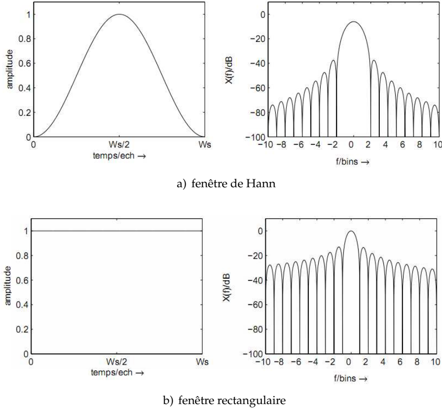
FIGURE 1.4 – Exemples de fenêtre d’analyse spectrale et spectre d’amplitude (en dB) correspondant [Mar08].
