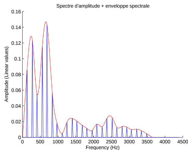
FIGURE 1.7 – Spectre d’amplitude d’un son de saxophone jouant la note \text{Do}\sharp_2 ( F_0 \approx 138.6\text{Hz} ). Nous voyons clairement les différents partiels (pics) ainsi que l’enveloppe spectrale correspondante (en rouge) construite par interpolation spline.
